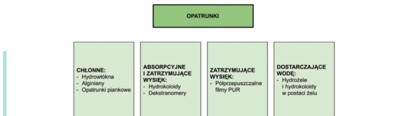
Rys. 3. Rodzaje opatrunków
