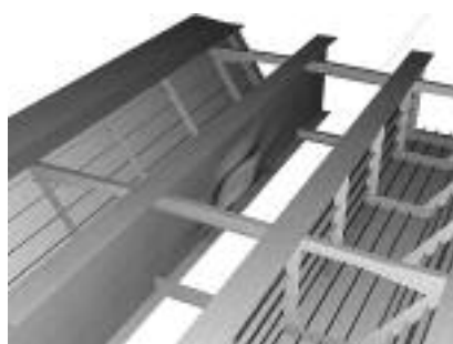
Rys. 9. Model szczegółowy, środniki bez wzmocnienia – postać wybożeniowa środnika wewnętrznego (mnożnik obciążenia przy wybożeniu wyniósł 1,01)
