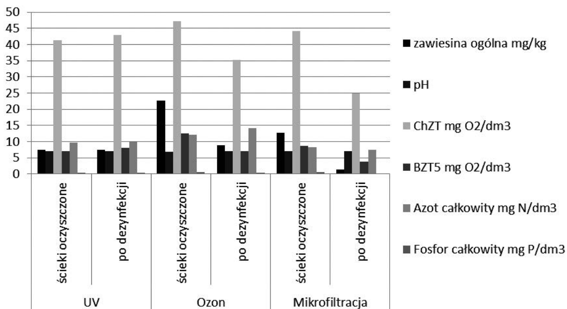
Rys. 4. Charakterystyka oczyszczonych i dezynfekowanych ścieków z OS „Wschód” w Gdańsku
