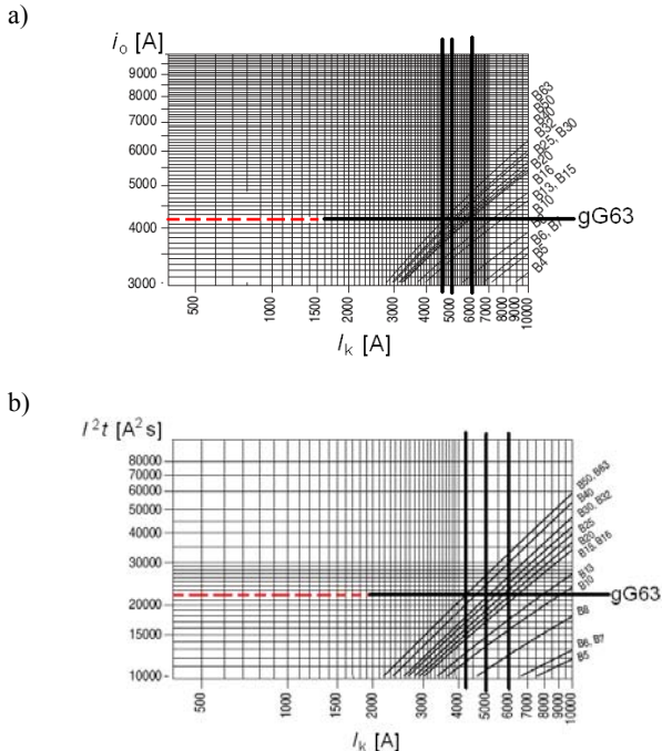
Rys. 6. Prąd ograniczony i_0 (a) i całka Joule'a wyłączenia I^2t_w (b) wyłączników nadprądowych instalacyjnych typu B [5]
