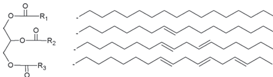
Rys. 2. Schematyczna struktura olejów roślinnych, R_1 , R_2 , R_3 – alifatyczne łańcuchy węglowodorowe kwasów tłuszczowych
