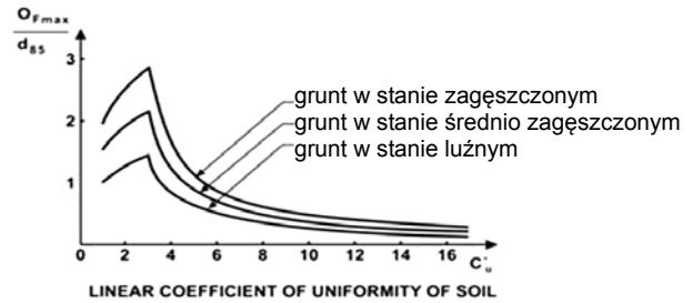
Rys. 2. Kryterium retencji z uwzględnieniem zagęszczenia i wskaźnika różnoziarności gruntu według J.P. Giroud [4]
