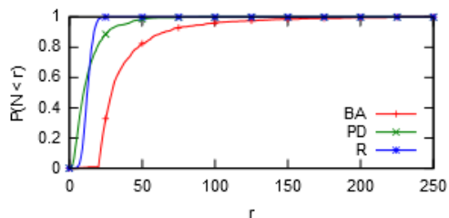
Rys. 1. Rozkład liczby węzłów sąsiednich
