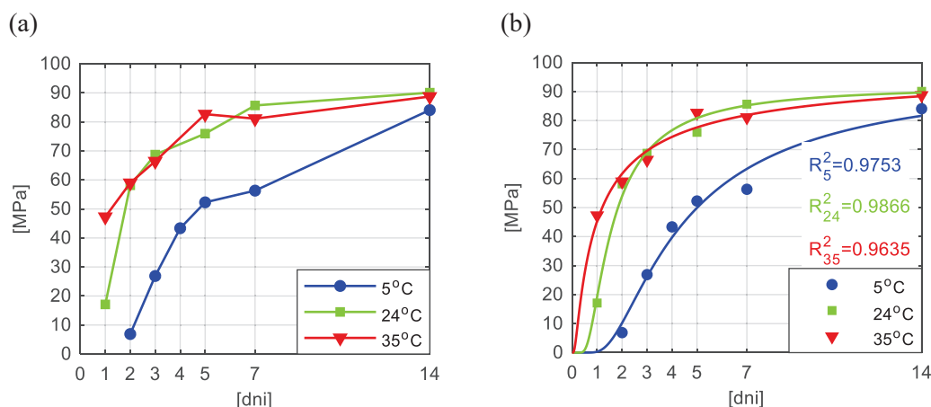
Rys. 5.6. (a) Średnia wytrzymałość zaprawy na ściskanie, (b) Aproksymacja danych wytrzymałościowych za pomocą funkcji eksponentialnej (3.23)
