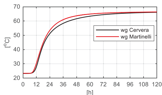
Rys. 6.13. Temperatura betonu w warunkach adyabatycznych według obu modeli
