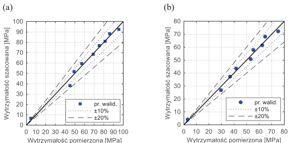
Rys. 5.22. Szacowana i pomierzona wytrzymałość betonu na ściskanie:
