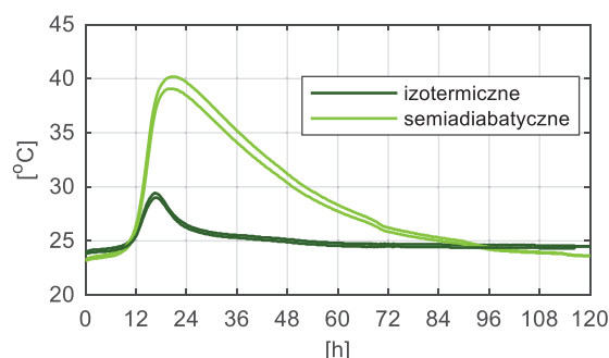
Rys. 6.9 Pomierzona temperatura betonu w warunkach izotermicznych i semiadiabacyjnych
