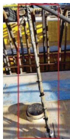
Rys. 5.33. (a) Widok płyty górnej, (b) Prefabrykowana listwa z czujnikami temp. zamocowana na pręcie
