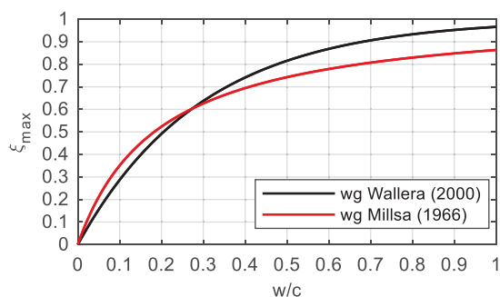
Rys. 6.4 Zależność finalnego stopnia hydratacji cementu od wskaźnika wodno-cementowego
