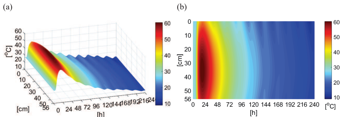
Rys. 6.24. Temperatura betonu płyty górnej: (a) rozkład, (b) mapa, (zmieniana temperatura otoczenia)
