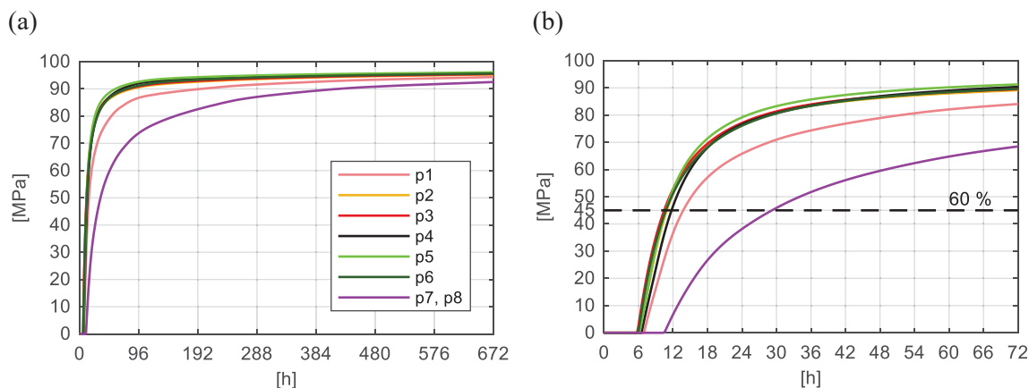
Rys. 5.23. Wytrzymałość kostkowa betonu płyty dolnej (wg p1 - p6) i próbek sześciennych (wg p7 - p8) w funkcji czasu: (a) 672 h=28 dni, (b) 72 h
