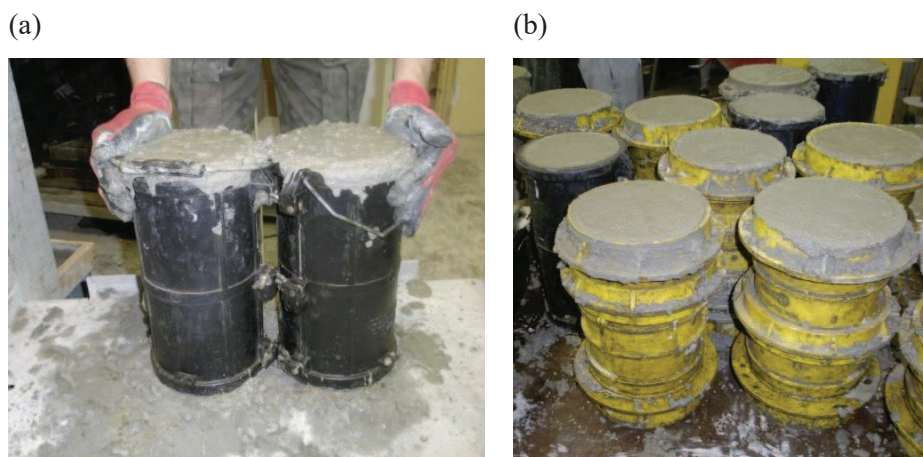
Rys. 4.2. (a) Zagęszczanie próbek na stoliku wibracyjnym, (b) Zaformowane próbki walcowe
