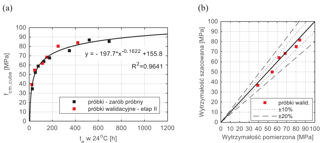
Rys. 5.36. (a) Krzywa dojrzłości betonu dla próbek sześciennych, (b) Pomierzona i szacowana wytrzymałość na ściskanie próbek sześciennych
