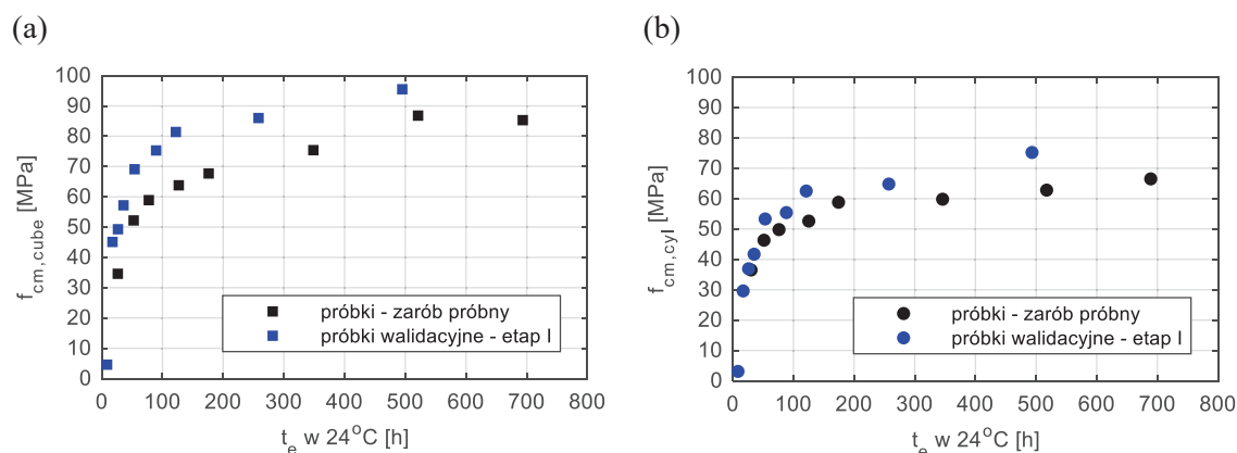
Rys. 5.20. Wytrzymałość na ściskanie w dziedzinie wieku równoważnego: (a) próbki sześciennie, (b) próbki walcowe
