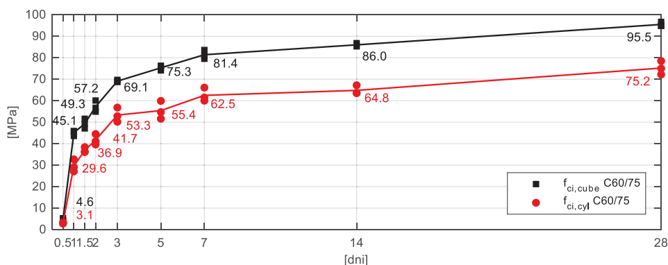
Rys. 5.19. Wytrzymałość na ściskanie walidacyjnych próbek walcowych i sześciennych
