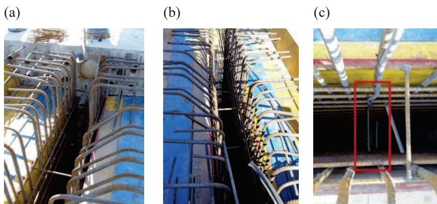
Rys. 5.27. (a), (b) Widok zazbrojonego środnika, (c) Czujniki temperatury w przekroju środnika
