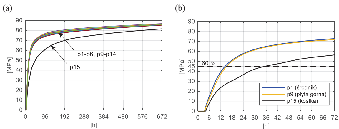
Rys. 5.38. Wytrzymałość kostkowa betonu środника i płyty górnej (wg p1 - p6, p9 - p14) oraz próbki sześcienniej (wg p15) w funkcji czasu: (a) 672 h=28 dni, (b) 72 h (wybrane punkty)
