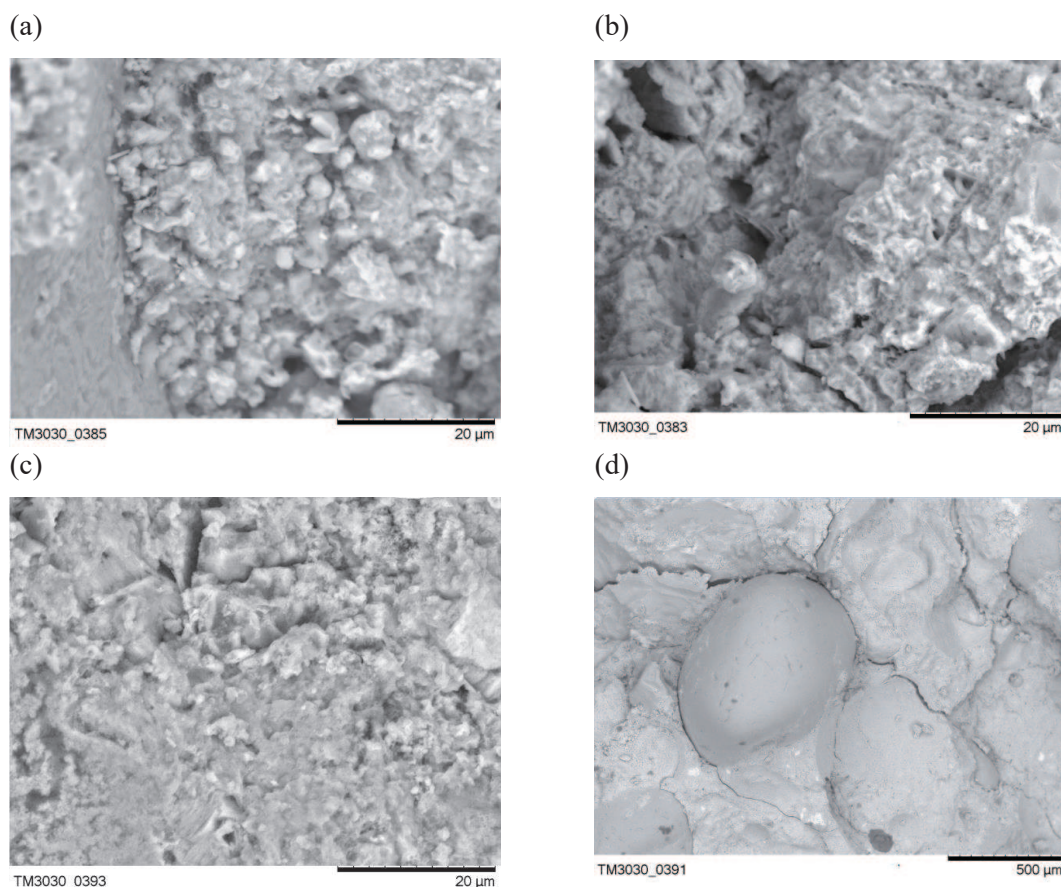
Rys. 4.12. Mikrostruktura zaprawy w powiększeniu do 20 μm dla próbek pielęgnowanych w temperaturze: (a) 9 °C, (b) 24 °C, c) 40 °C, (d) Widok na ziarno kruszywa (40 °C)
