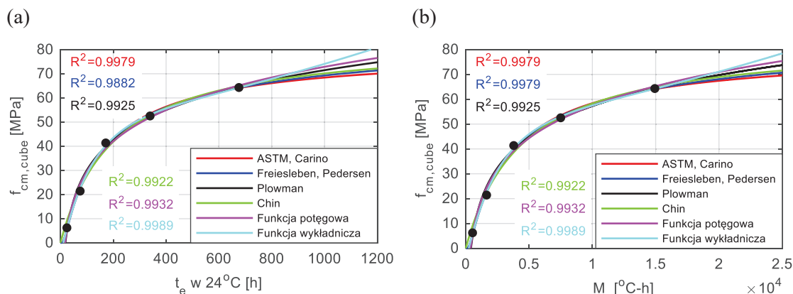
Rys. 4.38. Krzywe dojrzalsości betonu dla próbek sześciennych: (a) w dziedzinie wieku równoważnego, (b) w dziedzinie wskaźnika temperaturowo-czasowego
