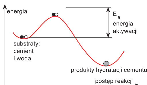
Rys. 3.3. Koncepcja energii aktywacji [89]
