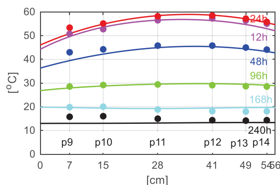
Rys. 6.25. Temperatura betonu w przekroju płyty górnej w wybranych godzinach (zmieniana, pomierzona temperatura otoczenia)
