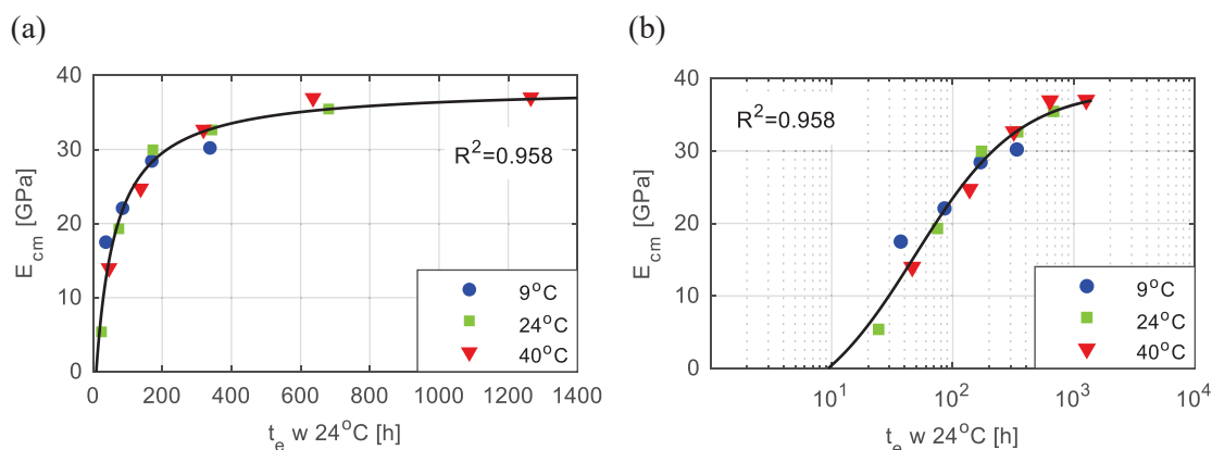
Rys. 4.45. Moduł sprężystości betonu w funkcji czasu równoważnego t_e : (a) skala liniowa, (b) skala logarytmiczna
