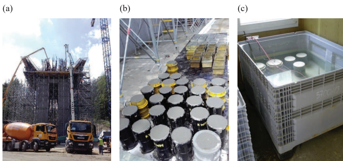
Rys. 5.15. (a) Betonownie płyty dolnej segmentu startowego, (b) Pobranie próbek do badań walidacyjnych, (c) Przechowywanie próbek i pomiar temperatury betonu
