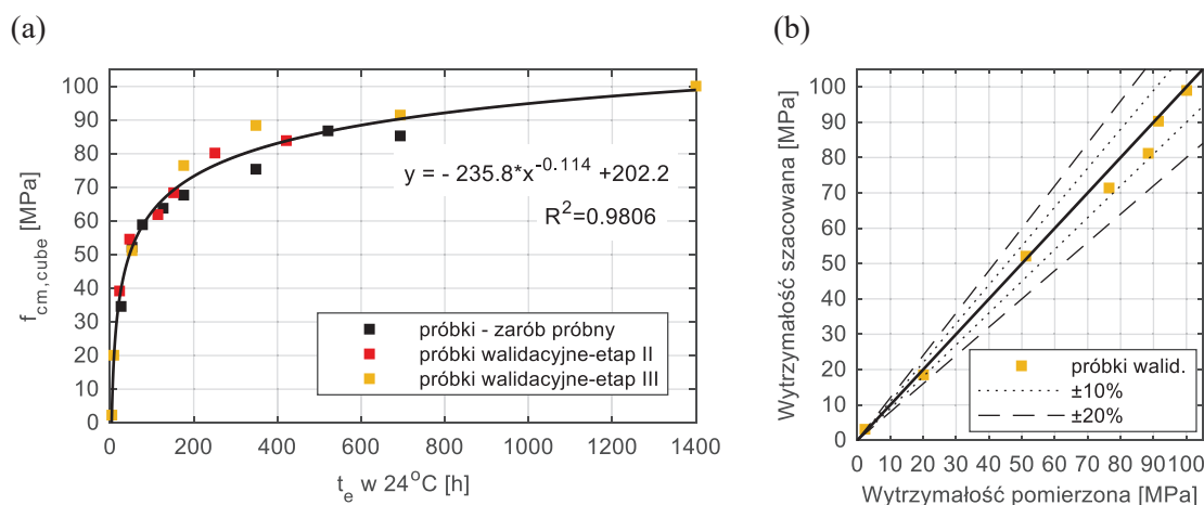
Rys. 5.50. (a) Krzywa dojrzłości betonu dla próbek sześciennych, (b) Wytrzymałość szacowana i pomierzona na próbkach walidacyjnych z etapu III
