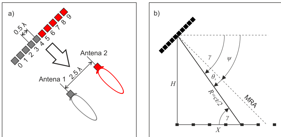
Rys. 7.3. Dynamiczne formowanie wiązek na przykładzie 10-elementowej anteny. a) Podział anteny odbiorczej na podanteny, b) Wyznaczanie kątów sterowania wiązek na podstawie wstępnego określania głębokości.
