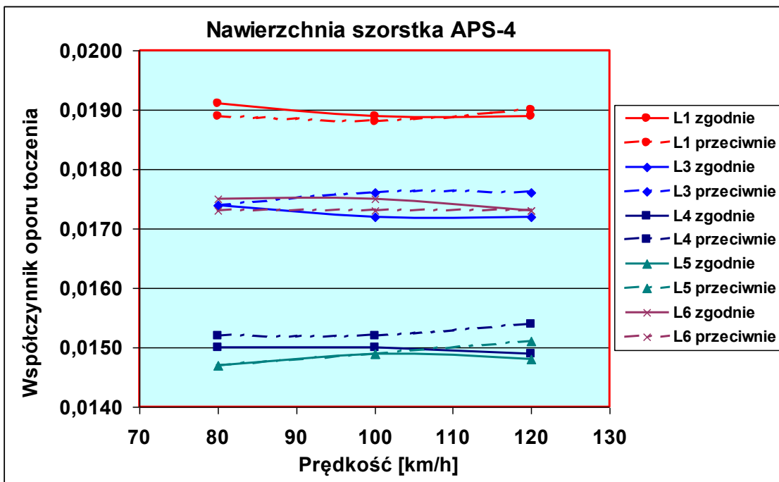
Rysunek 24. Opór toczenia opon kierunkowych z drogą rzeźbą bieżnika, toczonej zgodnie i przeciwnie do kierunku oznaczonego na oponie na nawierzchni APS-4 [2]
