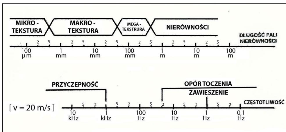
Rysunek 30. Częstotliwości odkształceń bieżnika opony w funkcji długości fali nierówności dla prędkości jazdy V=20\text{m/s} [28]
