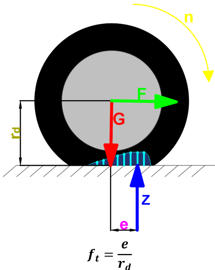
Rysunek 1. Schemat sił działających na toczące się koło samochodowe (materiał własny)
