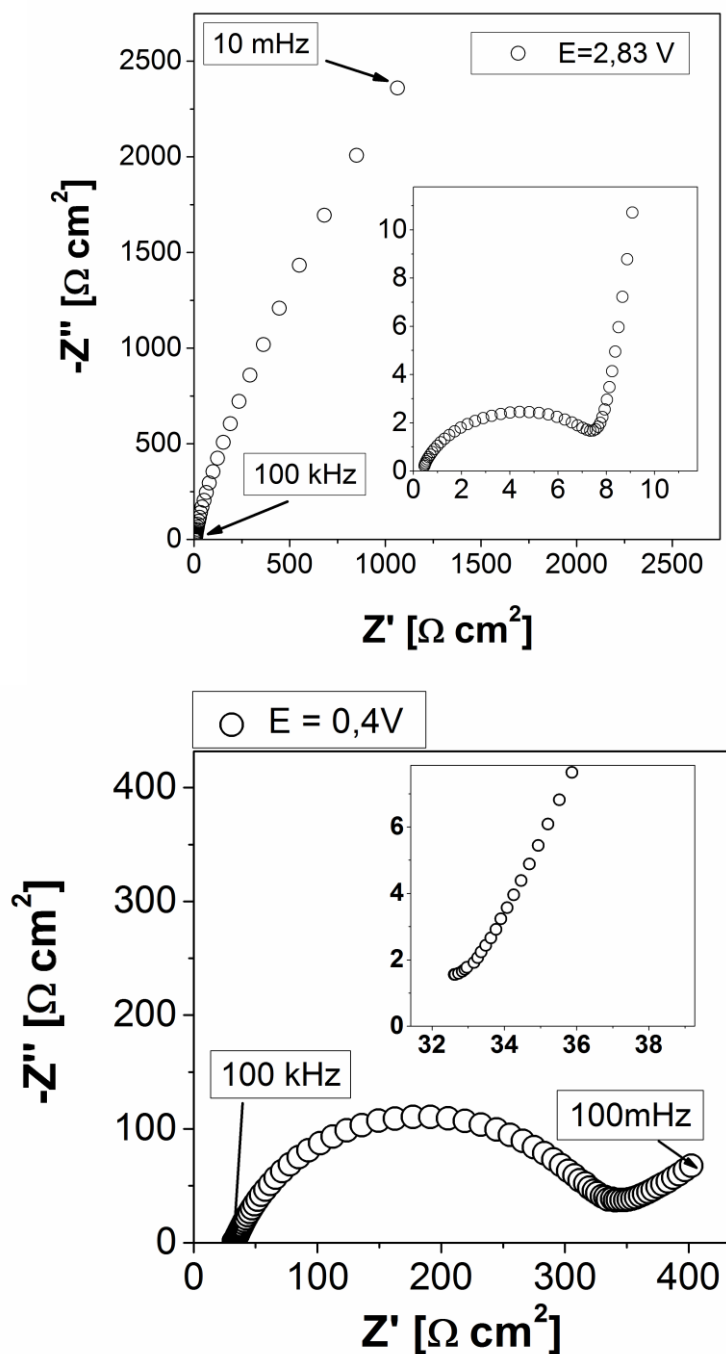
Rys. 42. Widmo impedancyjne dla elektrody Li||1 M LiPF 6 (EC:DMC)||ZO/CB/pVDF w zakresie częstotliwości od 1kHz do 10 mHz wykonana przy potencjale a) 2,83 V b) 0,4 V
