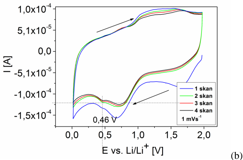
Rys. 57 Krzywe woltamperometrii cyklicznej dla materiału elektrodowego \text{SiO}_2@Cu/Cu_xO_y (a) w zakresie potencjałów od 0,02 – 3,10 V (vs. \text{Li/Li}^+ ) z szybkością skanowania 100 \mu\text{Vs}^{-1} (b) w zakresie potencjałów 0,02 - 1,95 V z szybkością 1\text{mVs}^{-1} [144].
