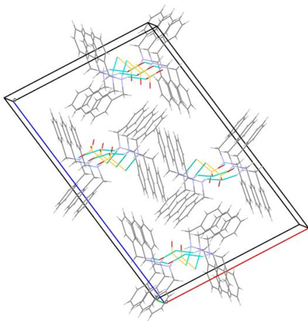
Rysunek 18. Upakowanie w kryształach tiosiarczanu bis(dibenzyloamoniowego) z widocznymi czterema prętami.
