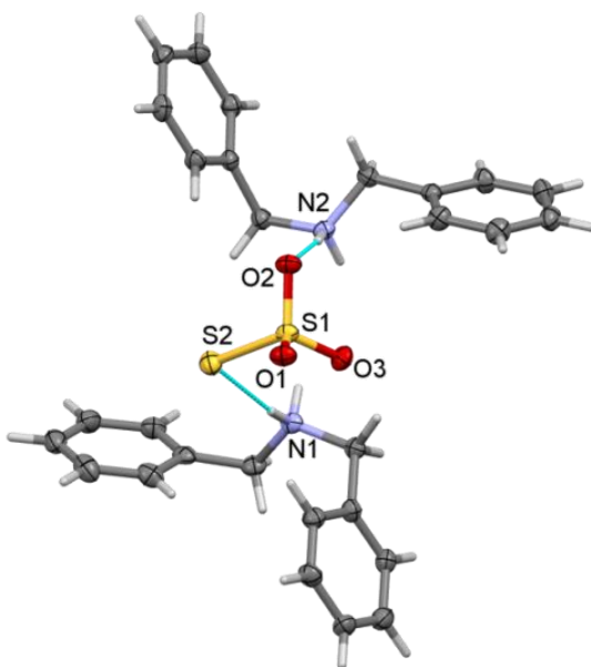
Rysunek 17. Struktura tiosiarczanu bis(dibenzyloamoniowego), elipsoidy drgań termicznych narysowane przy 50% poziomie prawdopodobieństwa.
