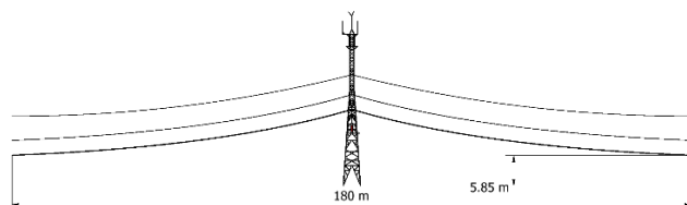
Rys. 2. Model geometryczny słupa PLN111 T w przęśle (wymiary charakterystyczne między punktami maksymalnego zwisu linii)
