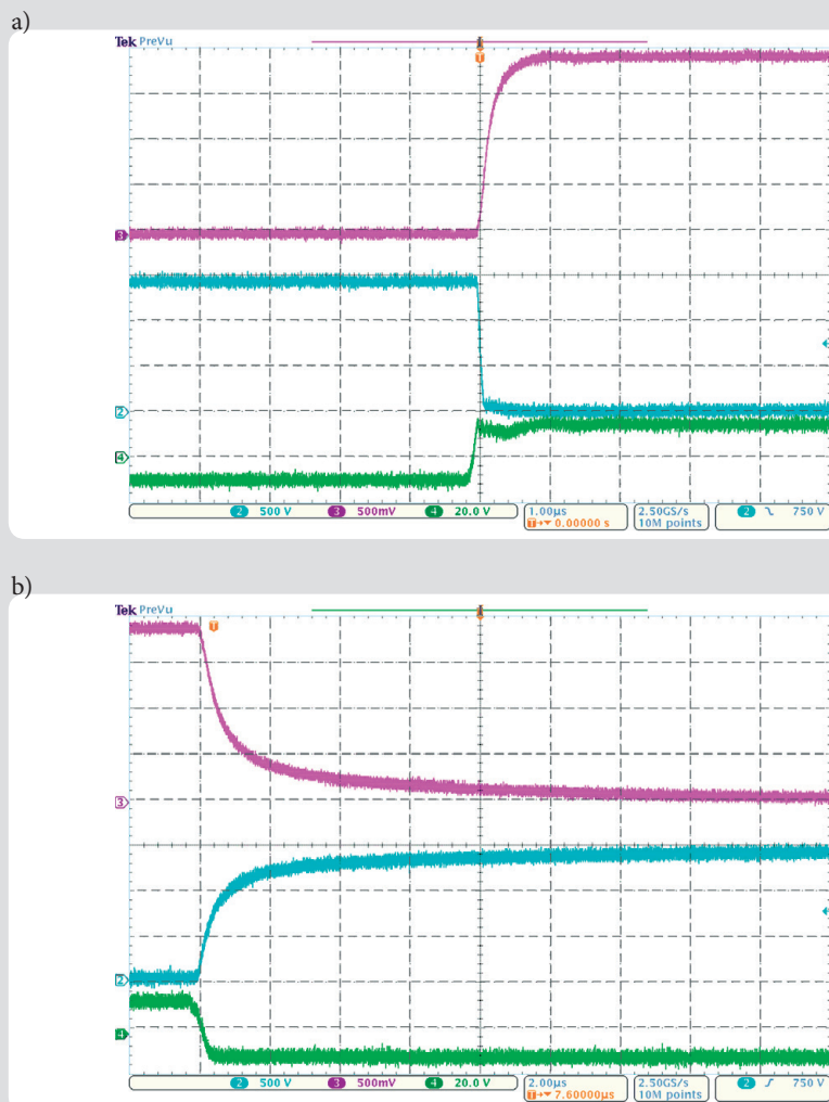
Rys. 4. Przebiegi uzyskane dla opracowanego półmostka IGBT w czasie załączania ( 1 \mu\text{s}/\text{dz} ) (a) oraz wyłączania ( 2 \mu\text{s}/\text{dz} ) (b) wysokonapięciowego tranzystora IXLF19N250A. Od góry: prąd ( 2,5 \text{ A}/\text{dz} ), napięcie na tranzystorze ( 500 \text{ V}/\text{dz} ) oraz napięcie na bramce ( 20 \text{ V}/\text{dz} )
