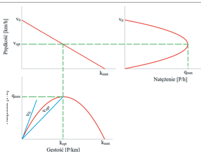
1. Przykładowy model zależności prędkość – gęstość – natężenie z oznaczeniem punktów charakterystycznych
