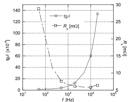
Rys. 4. Charakterystyki \text{tg}\delta i R_S w funkcji częstotliwości f pomierzone dla kondensatora typu MKSP-118 (7,5µF/425V) przy napięciu skutecznym polaryzacji 1V; pomiary wykonano mostkiem RLC GenRad 1689M
