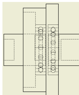
Rys.4. Rzut sprężła magnetycznego zaproponowanego do przeniesienia napędu
