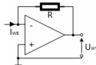
Rys. 4. Konwerter prąd-napięcie
