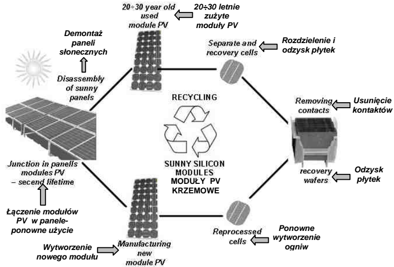
Rys. 6. Odzysk oraz ponowne wykorzystanie materiałów - krzemowych modułów PV Fig. 6. The recovery and renewed recycling of the materials - photovoltaic silicon modules
