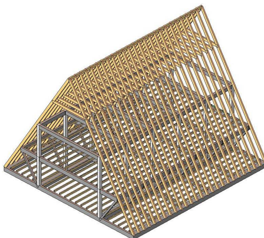
Rys. 9. Więźba dachowa z krokwiami ciągłymi z drewna klejonego o geometrii szkieletu żelbetowego z dodatkowym stropem i zastrzałem rygła pośredniego w połowie wysokości.
