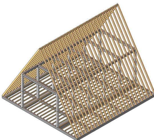
Rys. 10. Więźba dachowa z krokwiami ciągłymi z drewna klejonego wspartymi na ramach z drewna klejonego.
