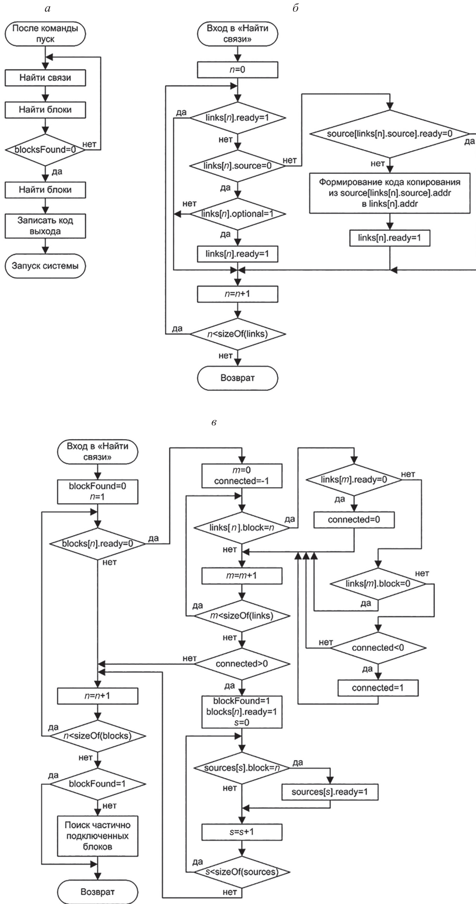
Рис. 5. Алгоритмы работы компилятора ядра системы управления: основной (а); поиска связей (б); поиска функциональных блоков (в)
