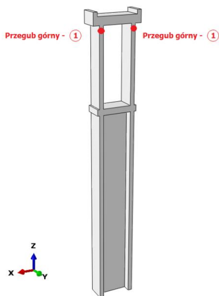
Rys. 79 Miejsce powstania przegubu plastycznego nr 1 (górnego) - Abaqus
