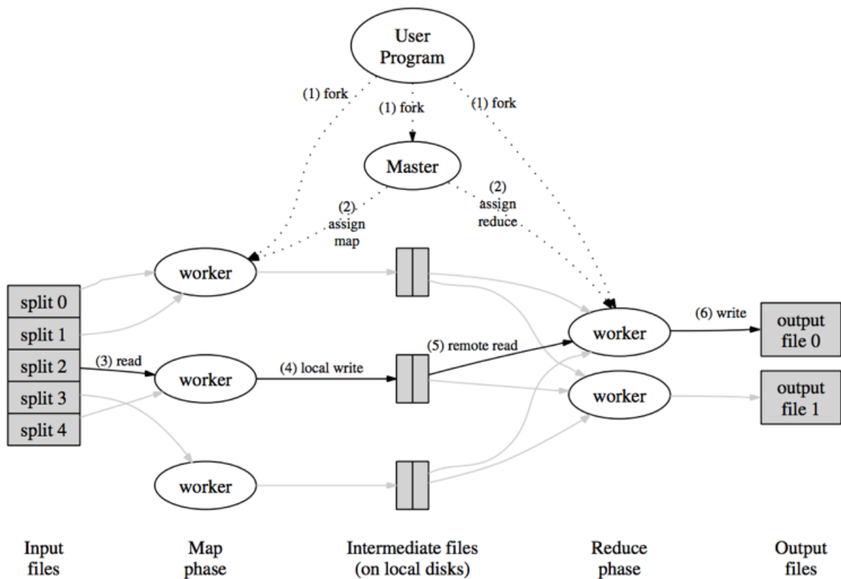
Rys. 2.10. Przykład działania modelu MapReduce [13].
