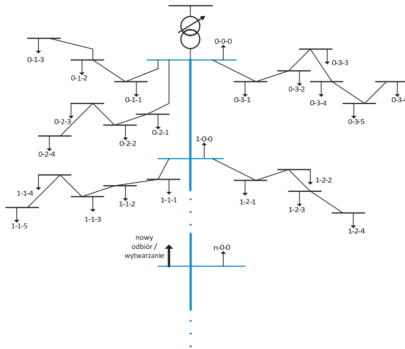
Rys. 1. Uproszczona struktura sieci promieniowej
