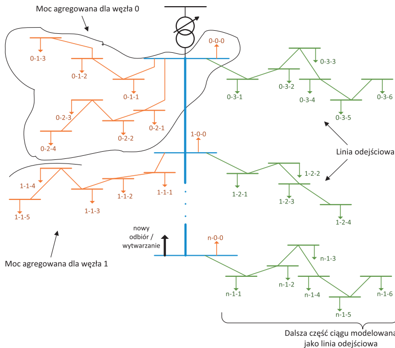
Rys. 2. Agregacja odgałęzień w sieci promieniowej
