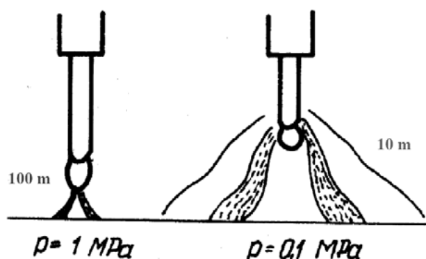
Rys. 3. Wpływ ciśnienia wody na zachowanie łuku elektrycznego [93]
