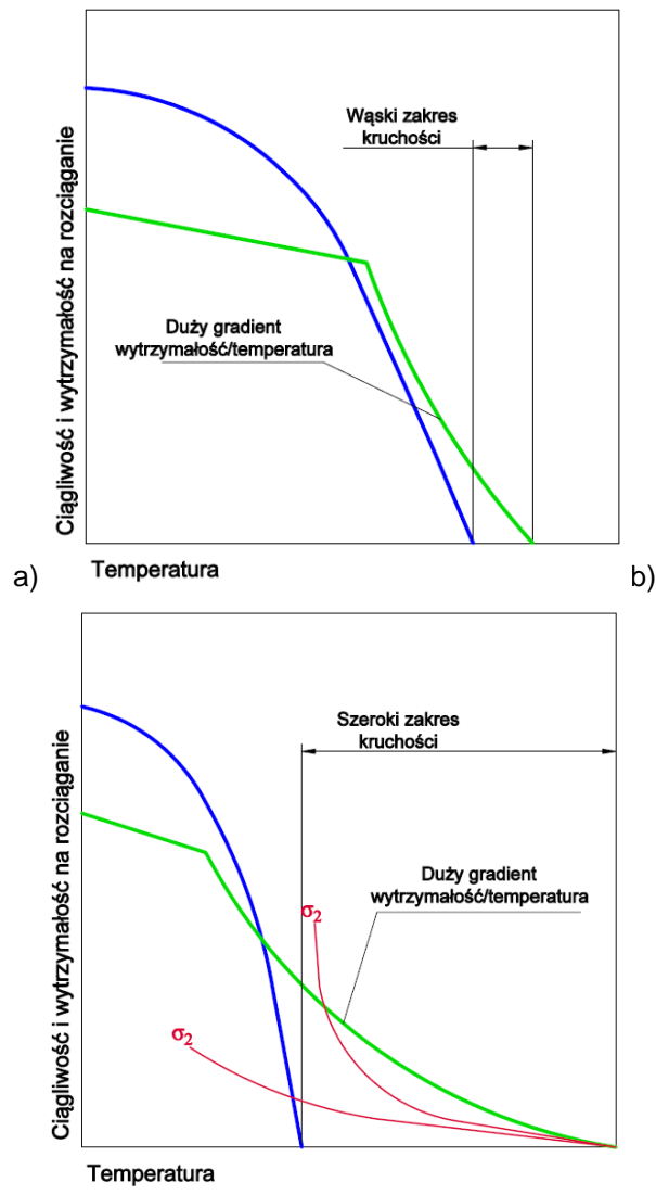
Rys. 34. Porównanie właściwości mechanicznych stopów w pobliżu linii solidus: a) metal odporny na pęknięcie, b) metal skłonny do pęknięcia; linia niebieska - ciągłość, linia zielona - wytrzymałość R_m , \sigma_1 i \sigma_2 - możliwe sposoby narastania naprężeń [18]
