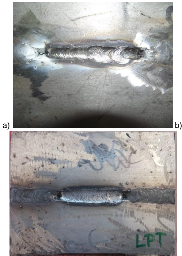
Rys. 105. Widok spoin próbnych w próbce TBP wykonanej elektrodami otulonymi Böhler (a) oraz próbki TLP wykonanej elektrodami Lincoln Electric (b) na powietrzu
