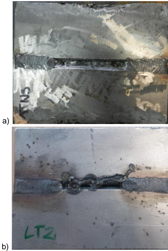
Rys. 104. Widok spoin próbnych w próbce 1TBM wykonanej elektrodami Böhler (a), oraz próbki LTM wykonanej elektrodami Lincoln Electric (b) w sztucznej wodzie morskiej
