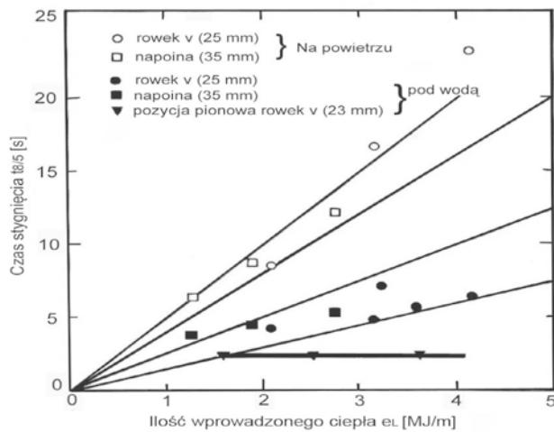
Rys. 2. Zależność czasu stygnięcia złącza od ilości wprowadzonego ciepła [6]: ○ – spawanie na powietrzu, ● – spawanie pod wodą, ◻ – napawianie a powietrzu, ◼ – napawianie pod wodą, ◆ – spawanie pod wodą w pozycji pionowej
