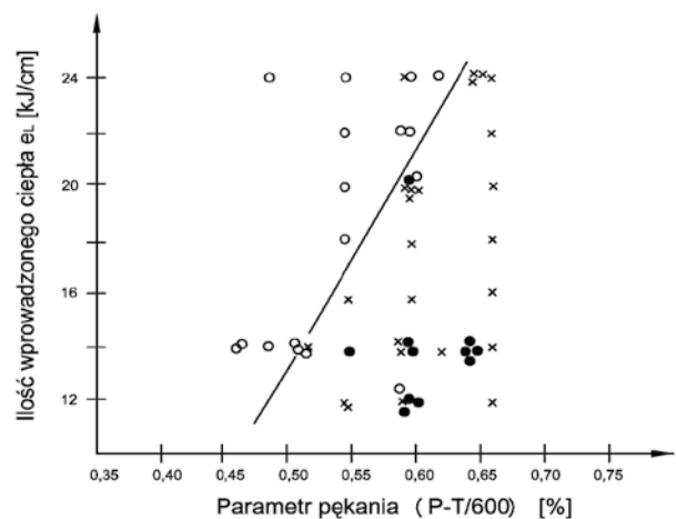
Rys. 4. Wyniki prób Tekken dla spawania mokrego MMA pod wodą [6]: ○ – brak pęknięć, × – pęknięcia wewnętrzne, ● – pęknięcia wewnętrzne i zewnętrzne
