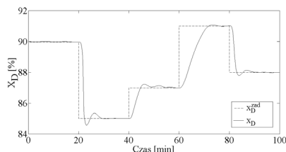
Rys. 10. Stężenie destylatu x_D Fig. 10. Distillate product composition x_D
