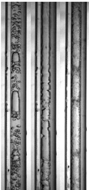
Rysunek 3: Struktury przepływu P_{zr}=0,2 G=355 \text{ kg}/(\text{m}^2\cdot\text{s}) stopnie suchości kolejno: 2%, 7%, 5,03%
