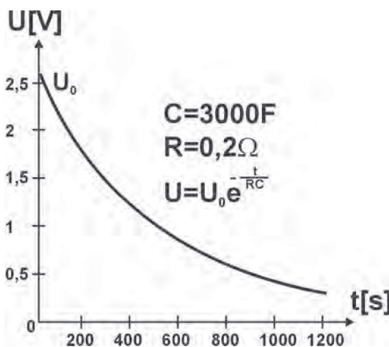
Fig. 2. Exemplary computer graph of a SC discharge U = f(t) curve, calculated and drawn with MATHCAD software. Rys.2. Przykładowy wykres komputerowy funkcji rozładowania U = f(t) superkondensatora, sporządzony za pomocą programu MATHCAD.
