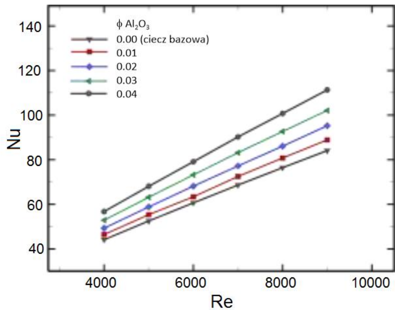
Rys. 4.17. Zależność liczby Nu od liczby Re dla nanocieczi woda- Al_2O_3 [108]
