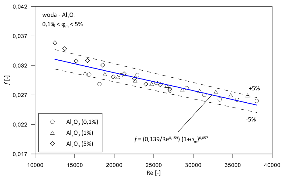
Rys. 7.21. Zależność f - \text{Re} dla nanocieczki woda- \text{Al}_2\text{O}_3
