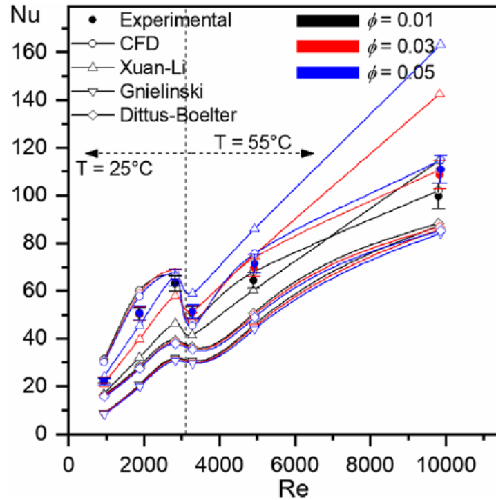
Rys. 4.16. Zależność liczby Nu od liczby Re dla nanocieczy woda-Al 2 O 3 [106]
