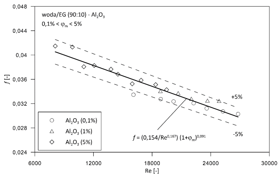
Rys. 7.22. Zależność f - \text{Re} dla nanocieczki woda/EG (90:10)- \text{Al}_2\text{O}_3
