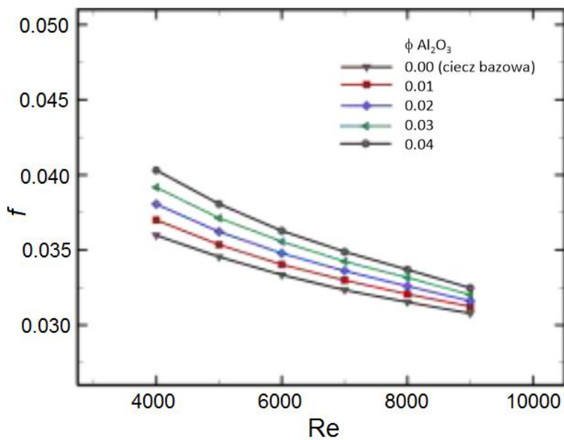
Rys. 4.18. Współczynnik oporów przepływu f dla nanocieczi woda- Al_2O_3 [108]
