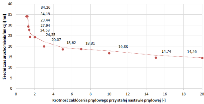
Rys. 10. Charakterystyka średniego czasu uruchomienia funkcji PHLPTOC w funkcji krotności wymuszenia zakłócenia względem nastawy prądowej przy stałej nastawie prądowej
