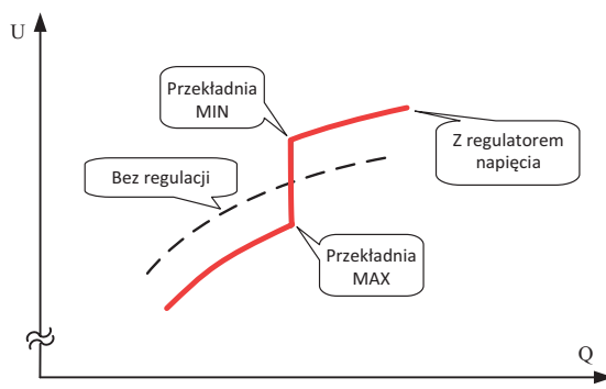
Rys. 4. Wpływ regulacji transformatora na charakterystykę Q = F(U) , uproszczenie: regulacja ciągła
