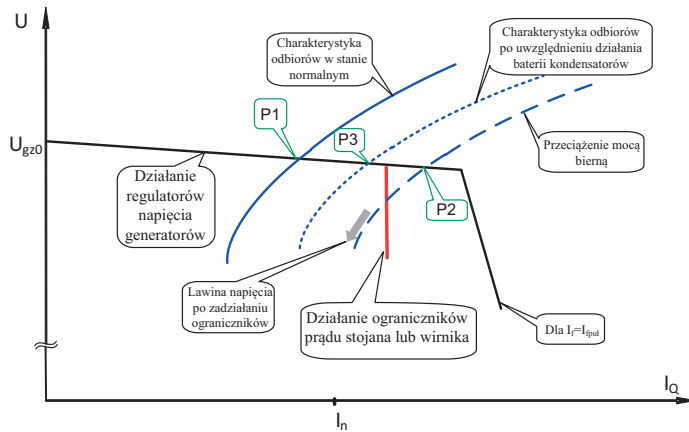
Rys. 3. Ilustracja wpływu działania lokalnej baterii kondensatorów w sytuacji wystąpienia deficytu mocy biernej
