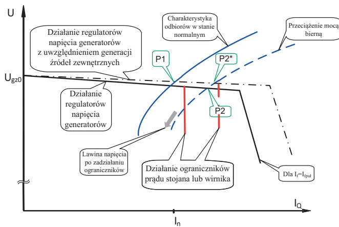
Rys. 2. Ilustracja wpływu lokalnej generacji w przypadku wystąpienia deficytu mocy biernej
