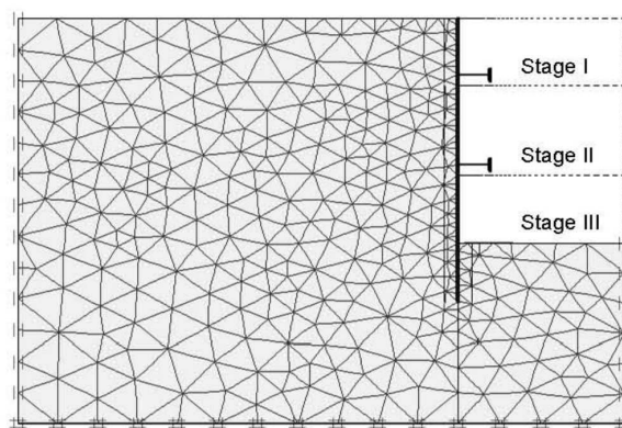
Fig. 4. Soil discretization by finite element mesh in PLAXIS program. Rys. 4. Podział ośrodka gruntowego na siatkę elementów skończonych w programie PLAXIS
