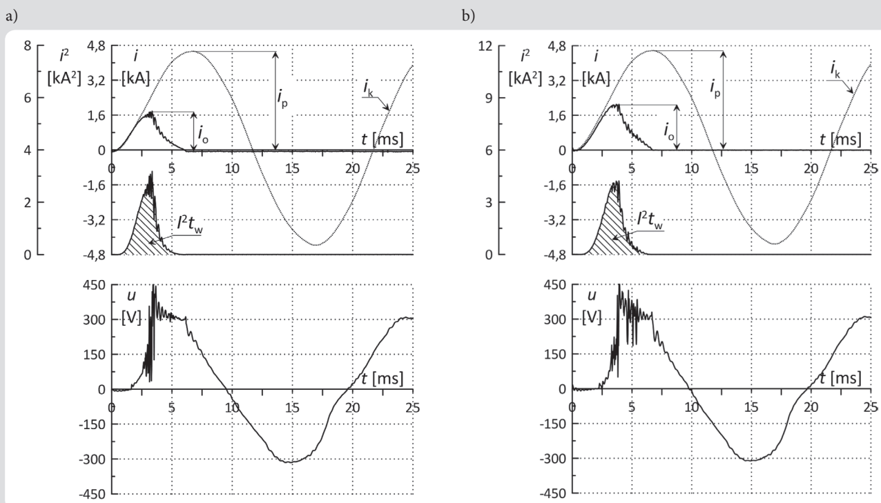
Rys. 3. Wyłączenie prądu zwarcia przez wyłącznik nadprądowy instalacyjny; I_k = 3,1 kA, i_p = 4,5 kA, a) wyłącznik C16, i_o = 1,8 kA, I^2 t_w = 4,8 kA 2 s, b) wyłącznik D20, i_o = 2,1 kA, I^2 t_w = 7,9 kA 2 s
