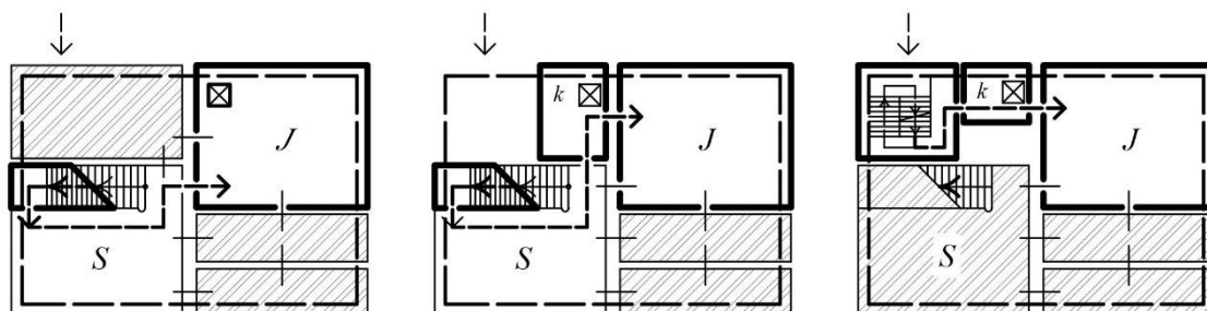
Schemat 3. Przykłady układu komunikacyjnego między jadalnią a piwnicą (kuchnia lokalizowana w piwnicy) J-jadalnia, S-sień, k-kredens; przykład pierwszy – najbardziej niekorzystny, przykład drugi – pośredni, przykład trzeci-komunikacja służby całkowicie uniezależniona od ogólnodostępnych ciągów komunikacyjnych.
