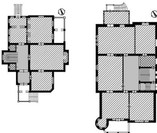
il. 87. Rzut parteru willi, w typie A-s (po lewej ul. Sternicza 2) i typie A-c (po prawej ul. Batorego 5). Wariant pierwszy komunikacji, w którym służba przemieszcza się za pośrednictwem głównego holu. Hol ten pełni również funkcję reprezentacyjnego westybulu.
