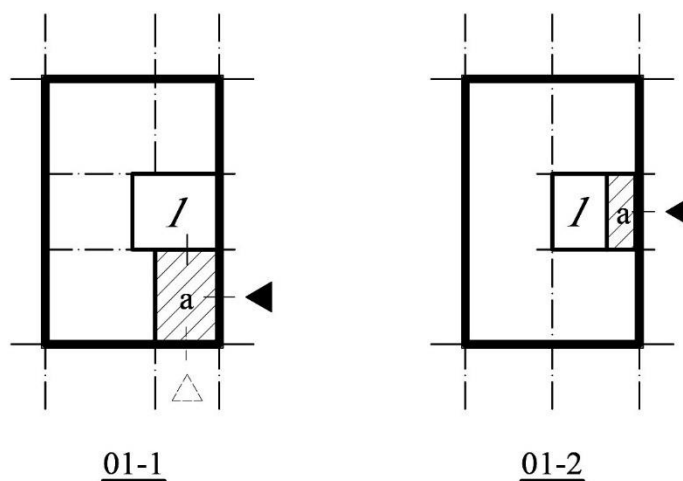
Schemat 10. Lokalizacja wiatrołapu i sieni w kontekście siatki konstrukcyjnej (I- sień, a – wiatrołap). Przykład rozwiązania 01-1 – plebania przy ul. Sobótki 20, willa przy ul. Sternicznej 2 (TYP 1-malowniczy), rozwiązania 01-2- np. Ul. Batorego 5 (TYP 2- malowniczy zwarty).
