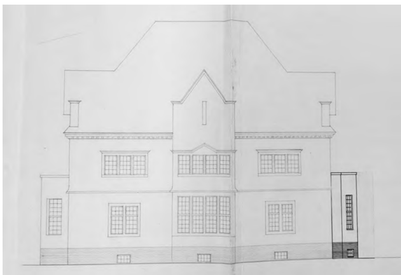
Elewacja boczna.
