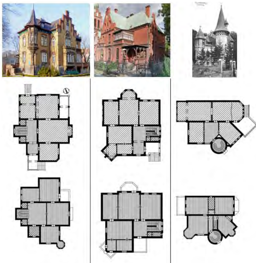
il. 83. Przykładowe rozwiązania dla willi w typie 1 - rozczłonkowanie bryły poprzez wielość rozwiązań formalnych (ryzality, wykusze, balkony, loggie, wykusze narożne, tarasy, ganki – widoczne w różnicach obrysach murów zewnętrznych parteru i piętra (od lewej: ul. Sternicza 2, ul. Sobótki 20, ul. Pawłowskiego 2).
