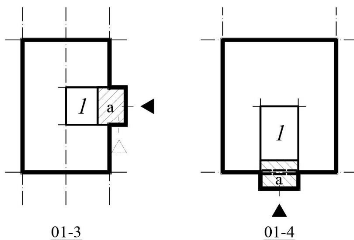
Schemat 11. Lokalizacja wiatrołapu i sieni w kontekście siatki konstrukcyjnej (I- sień, a – wiatrołap). Przykład rozwiązania 01-3 – ul. Jaśkowa Dolina 47 (TYP 3-zwarty, uproszczony), rozwiązanie 01-4 – ul. Polanki 115 (TYP 4 – landhaus).
