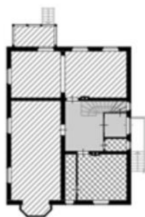
il. 85. Przykład zabudowy w typie 3. Od lewej - wariant 31- ul. Uphagena 7, wariant 33 – ul. Batorego 20, wariant 34- ul. Uphagena 30 (nieistn.)
