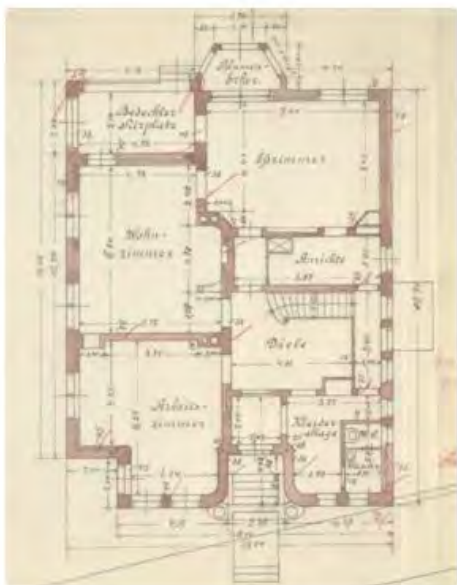
il. 88. Rzut parteru willi w typie B podłużnym -(po lewej ul. Batorego 10, po prawej ul. Sobótki 18). Oba projekty autorstwa Alberta Carstena przedstawiają aranżację, w której komunikacja między kondygnacją suterenu a parterem odbywa się niezależnie od sieni, która w tym wypadku może nabrać cech pomieszczenia dziennego (Diele).
