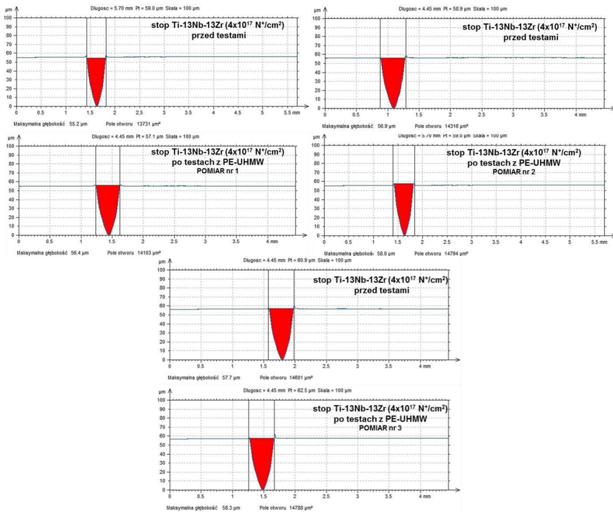
Rys. 123. Wyniki pomiarów głębokości rowków obwodowych oraz pola powierzchni rowków przed i po testach tribologicznych dla próbki ze stopu Ti-13Nb-13Zr ( 4 \times 10^{17} N + /cm 2 ) współpracującego z PE-UHMW
