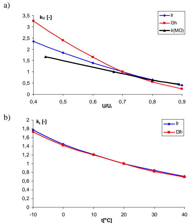
Rys. 3. Współczynniki poprawkowe [5, 6]– a) wpływu napięcia, b) temperatury do przeliczenia pomiarów prądu upływowego na warunki odniesienia – 20°C i U/U_r=0,7
