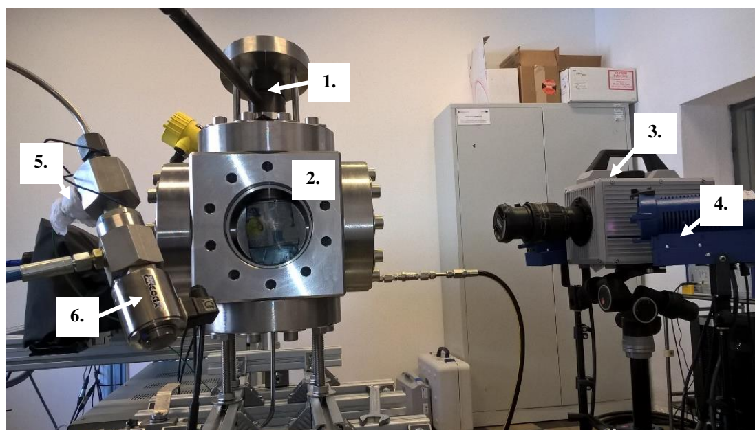
Rys. 3.3 Stanowisko pomiarowe metody optycznej techniką Mie scattering:
