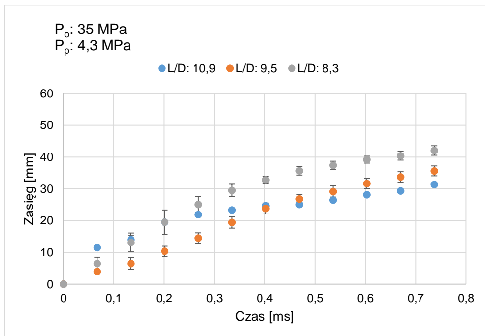
Rys. 5.14 Zasięg strugi rozpylanego oleju napędowego dla P_o : 35 MPa, oraz P_p : a. 3,2 MPa, b. 4,3 MPa
