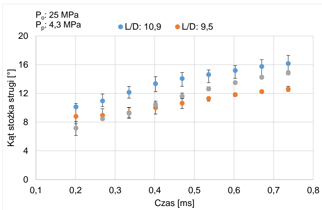
Rys. 5.7 Kąt stożka strugi dla P_0: 25 \text{ MPa} , oraz P_p : a. 3,2 MPa, b. 4,3 MPa
