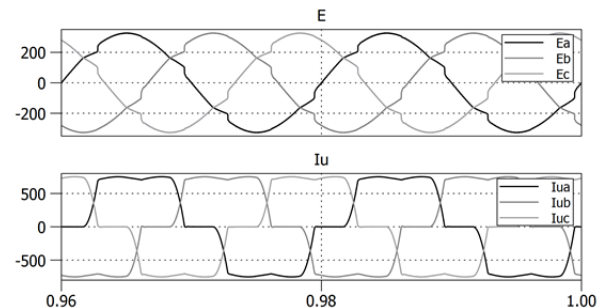
Rys.4. Brak kompensacji harmonicznych; L_s=40 \mu\text{H} ; \text{THD}_i=5,1 \% , \text{THD}_v=24 \%
