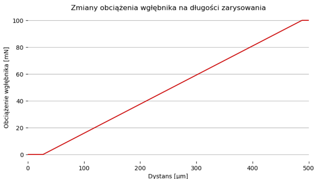
rys. 10.3. Zmiany obciążenia wgłębnika w czasie testu zarysowania powłoki.
