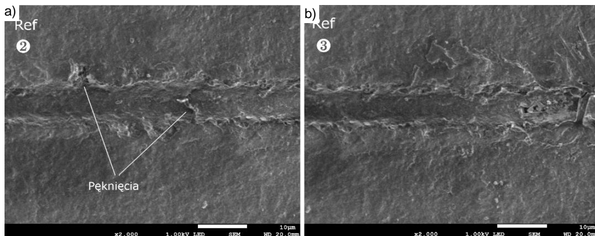
rys. 11.13. Powiększone fragmenty zarysowania powłoki referencyjnej, w których: pojawiły się pęknięcia – rys. a) oraz wykruszenia powłoki na dnie zagłębienia – rys. b).
