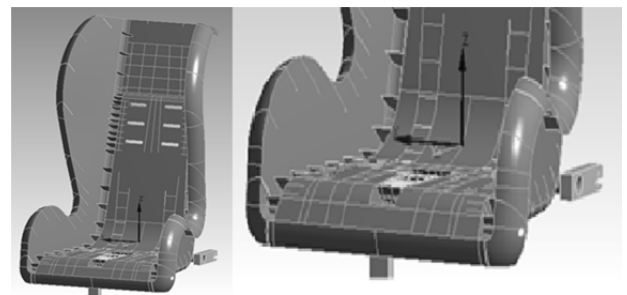
Rys. 4. Globalny układ odniesienia przyjęty do obliczeń [1]
