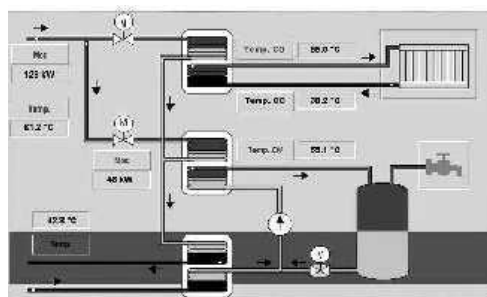
Rys. 2. Aplikacja wizualizacyjna funkcji SCADA [3]
