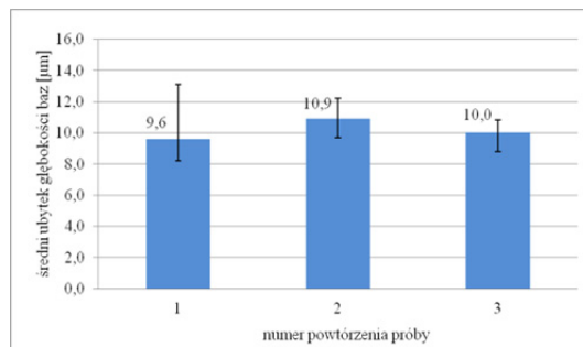
Rys. 15. Wyniki badań zużycia pierścieni prowadzących w doświadczeniu 3 (mikroziarnami 95A F600, \omega_1 = 6,28 rad/s, \omega_2 = 5,87 rad/s, v_d = 7,66 m/min)
