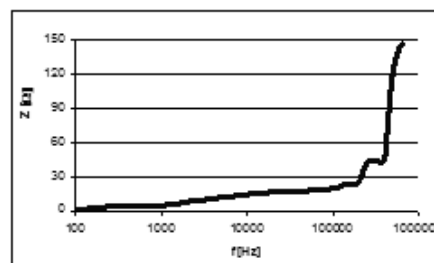
Rys. 5. Wartość impedancji uziemia słupa linii przesyłowej wysokiego napięcia w funkcji częstotliwości wyznaczona miernikiem AES 1002 Fig. 5. Earthing impedance of transmission line tower vs frequency, tests performed with use of AES 1002 meter
