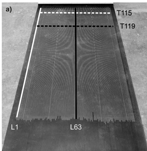
Rys. 4. Trasy wykonywanych skanów: a) badanie nr 1: skany podłużne z użyciem maty PSG; b) badanie nr 2: skany podłużne i poprzeczne bez użycia maty PSG
