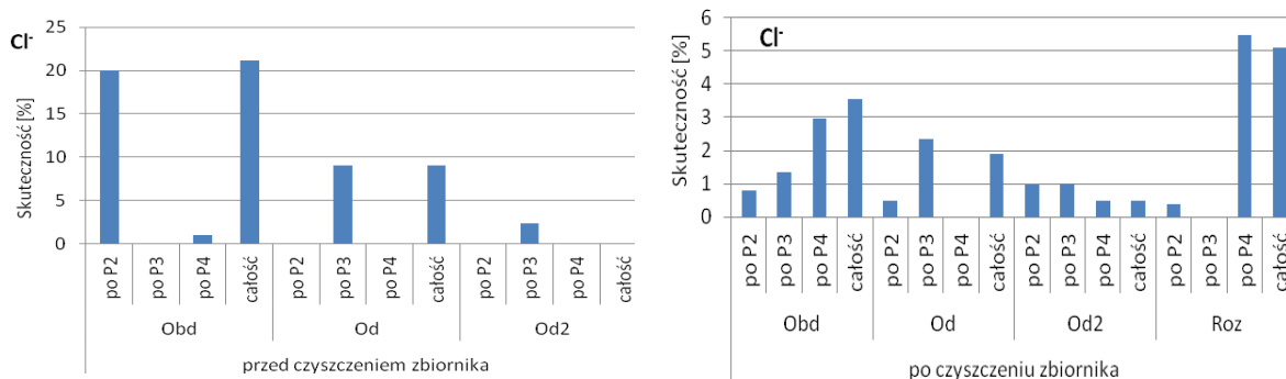
Rys. 5.28. Skuteczność usuwania chlorków po kolejnych stopniach czyszczenia
