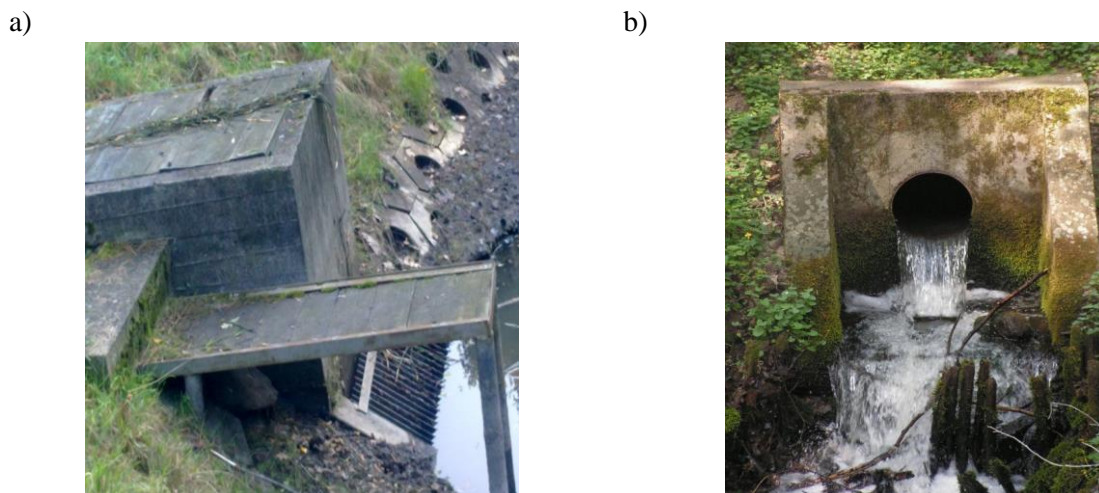
Rys. 3.11. Widok na: a) przelew do złoza hydrofitowego i b) odpływ ze studni kontrolnej po złożu hydrofitowym (fot. Marzena Stosik)
